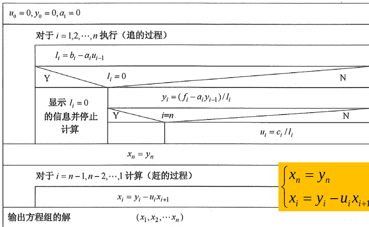
图 4.4.1 追赶法的算法框图
