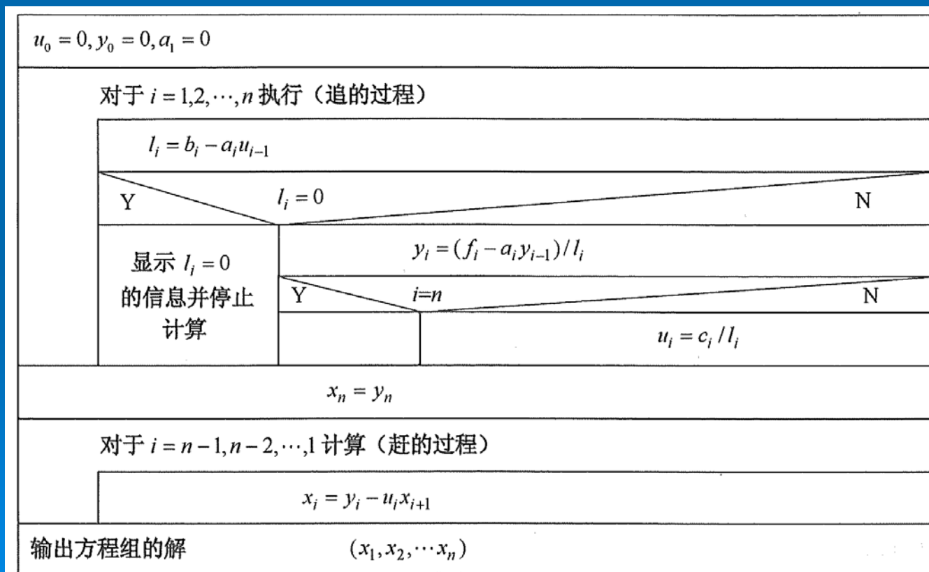
图 4.4.1 追赶法的算法框图
