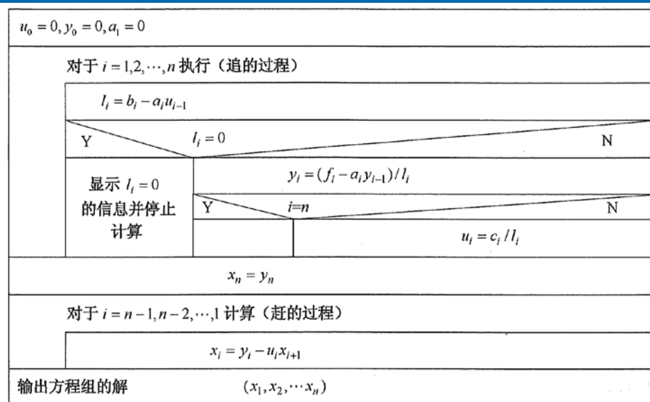
图 4.4.1 追赶法的算法框图
